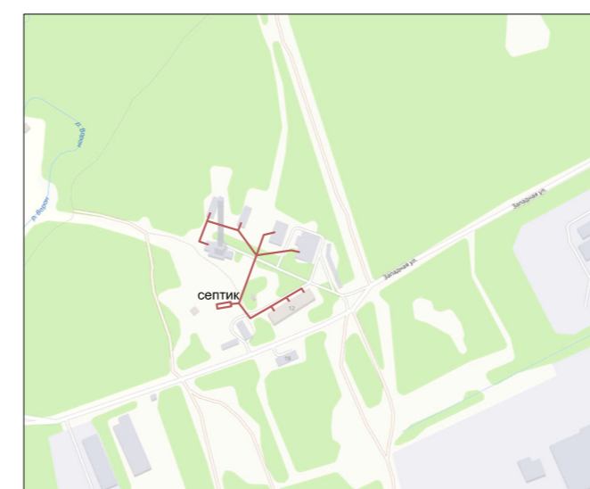
Схема водоотведения ул. Западная
