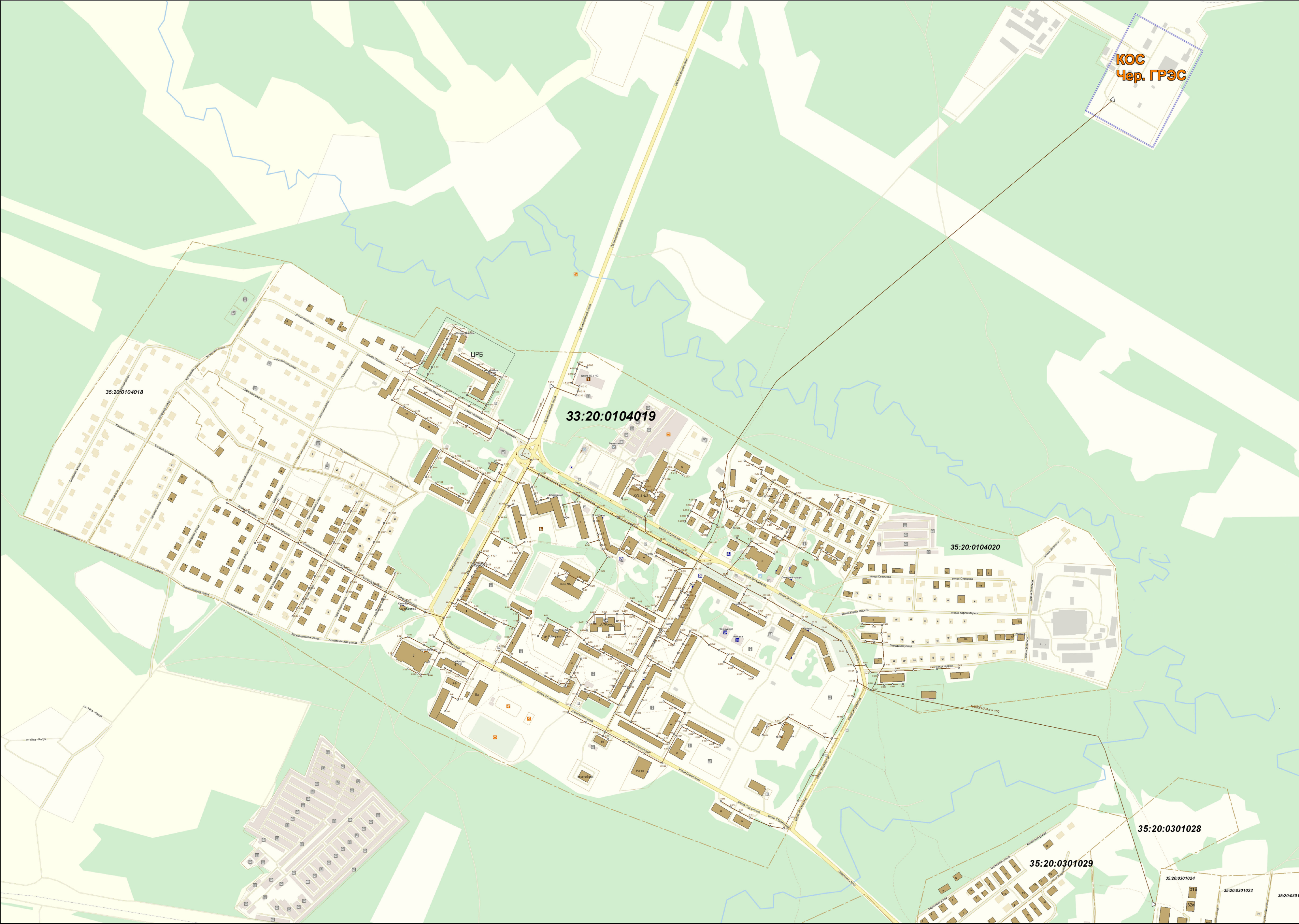
Схема водоотведения п. Кадуй
